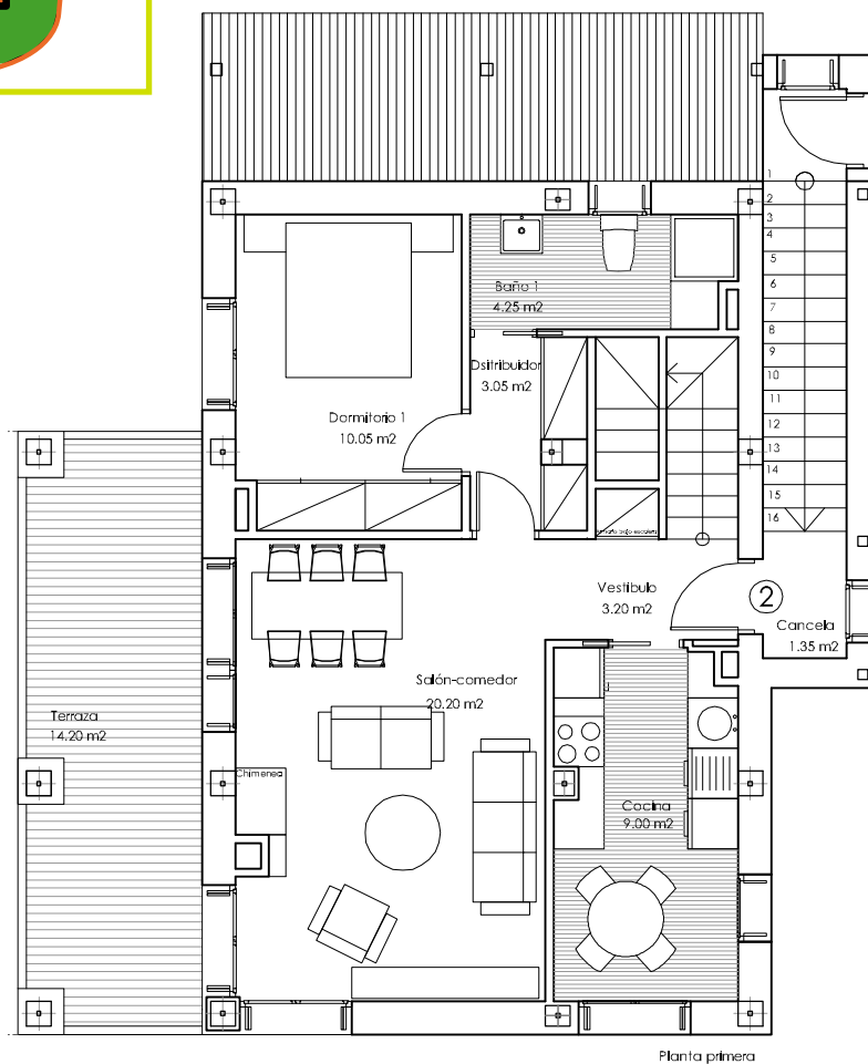
Planta primera
